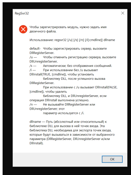
Рисунок 8 – Окно RegSvr32
